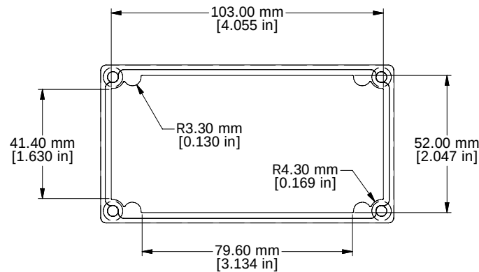
DEEP LID - INSIDE
