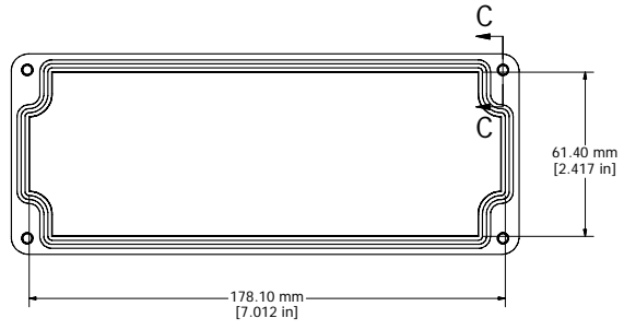
LID - INSIDE
