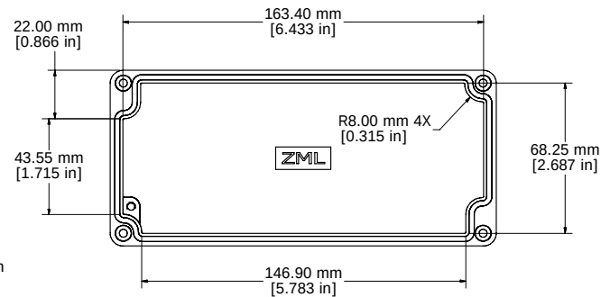
LID - INSIDE
